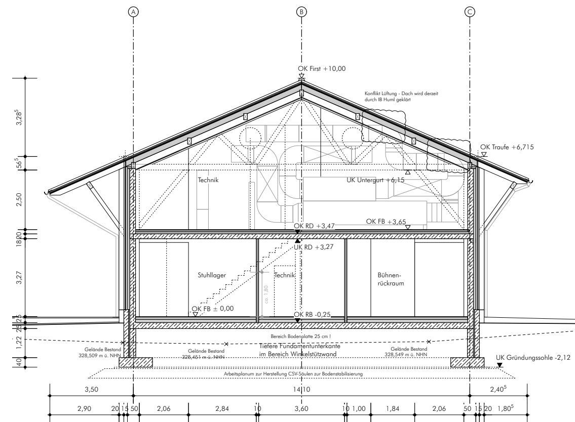
Schnitt C-C
