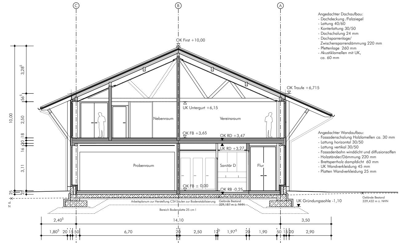
Schnitt B-B
