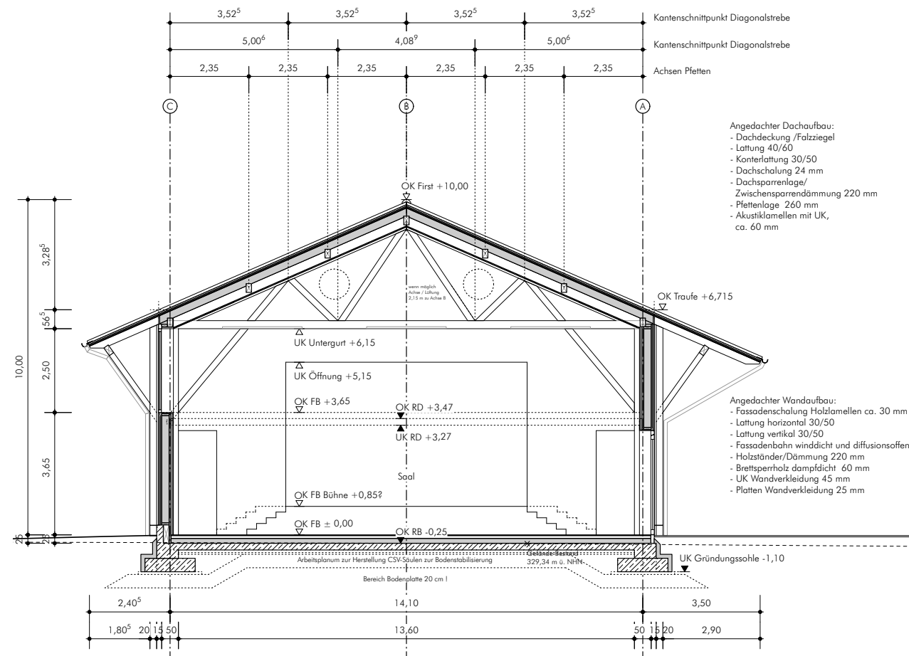
Schnitt A-A
